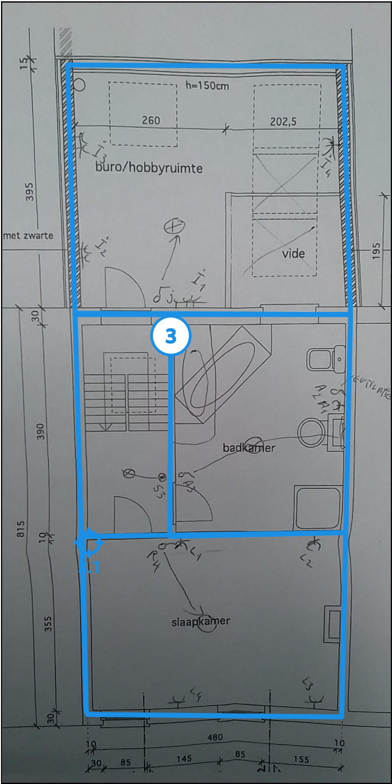
Legende van plan 1.3: Verdiep +1 : pleisterwerk wanden
