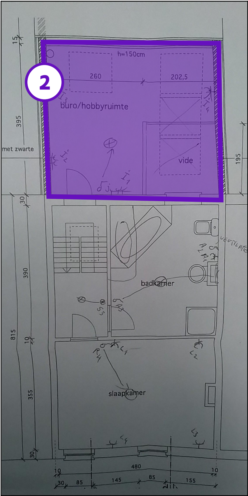
Legende van plan 1.5: Verdiep +1 : vals plafond
